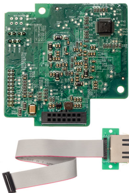
PD310PN1 Модуль Profinet
